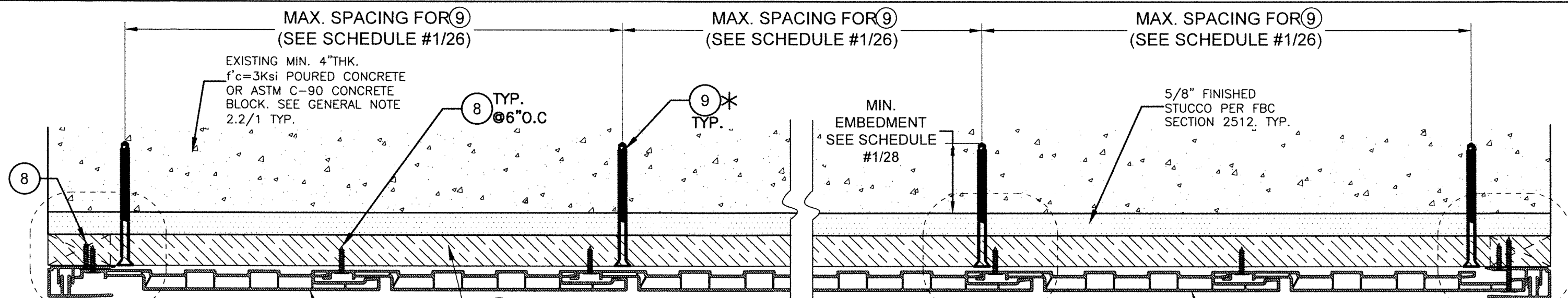
SECTION A-A SCALE: N.T.S
